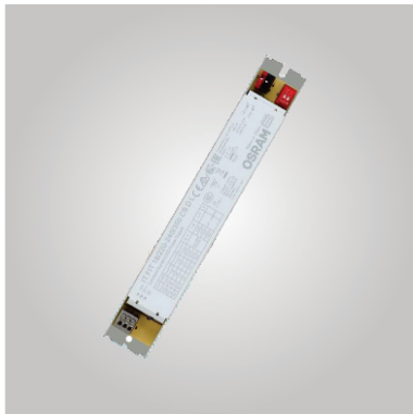
FPC NTO-18 Ersatznetzteil 18 W / 350 mA
